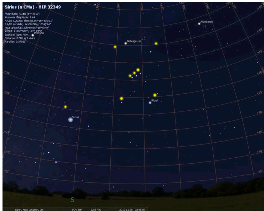
Fig 24: Sterrenhemel op 28 november 2010 om 2u45 met duidelijk zichtbaar de drie sterren van de Oriongordel, Sirius, Rigel en Betelgeuze. De gele punten zijn de stationaire objecten zoals die door de getuige werden getekend. De overeenkomst met de posities van de sterren is frappant. © Stellarium
