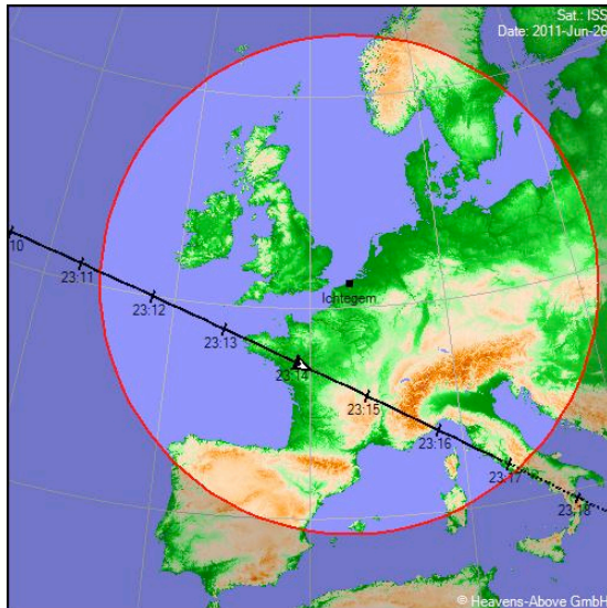
Fig 56: Traject van het ISS (bron: www.heavens-above.com )
